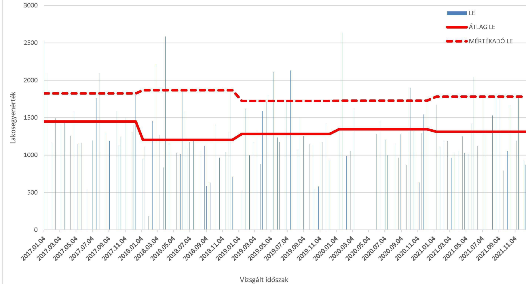
3.2. ábra_2017-2021. évi szennyvízterhelési adatok
