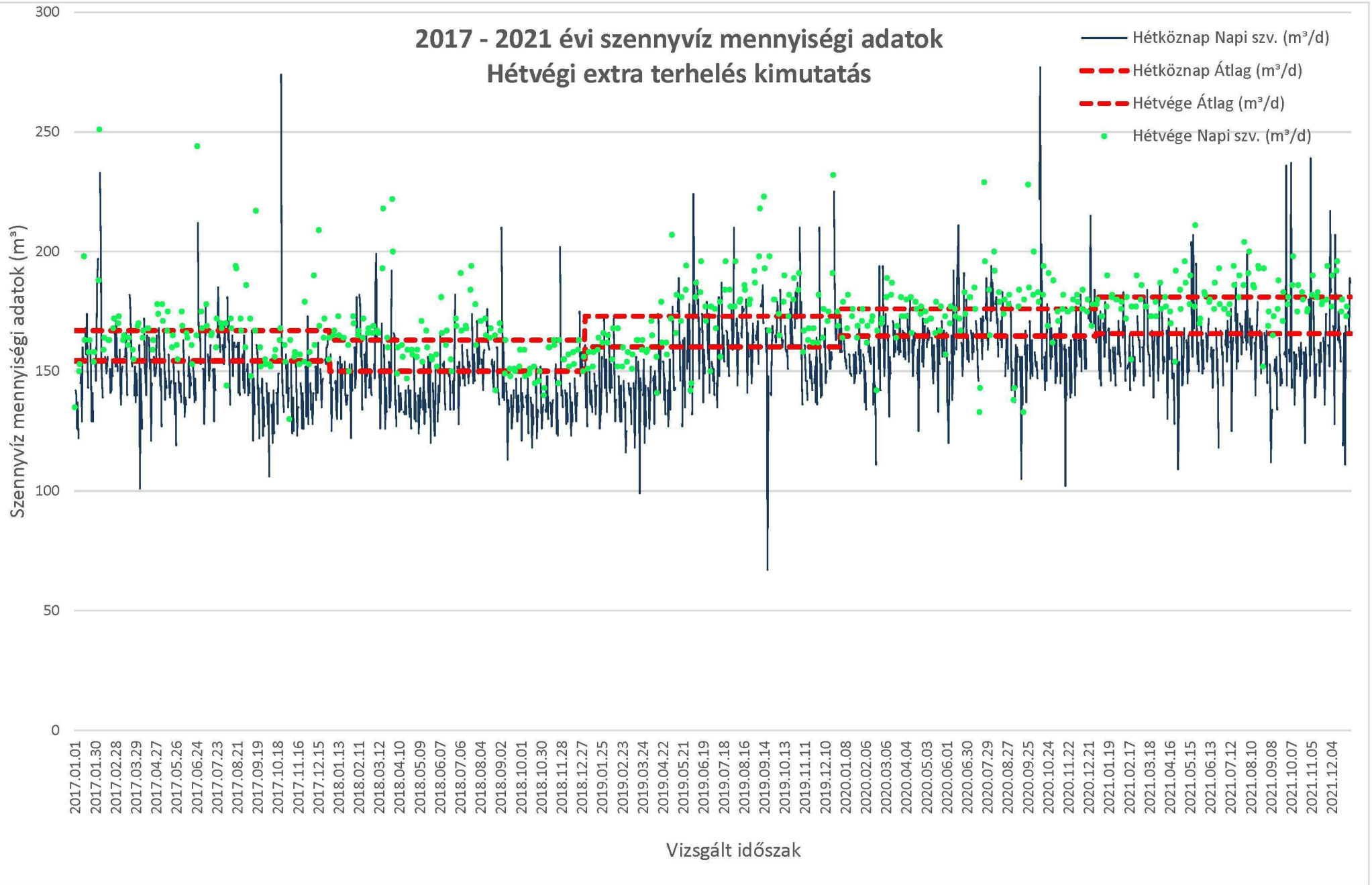
3.3. ábra_2017 - 2021 évi szennyvíz mennyiségi adatok Hétfégi extra terhelés kimutatás
