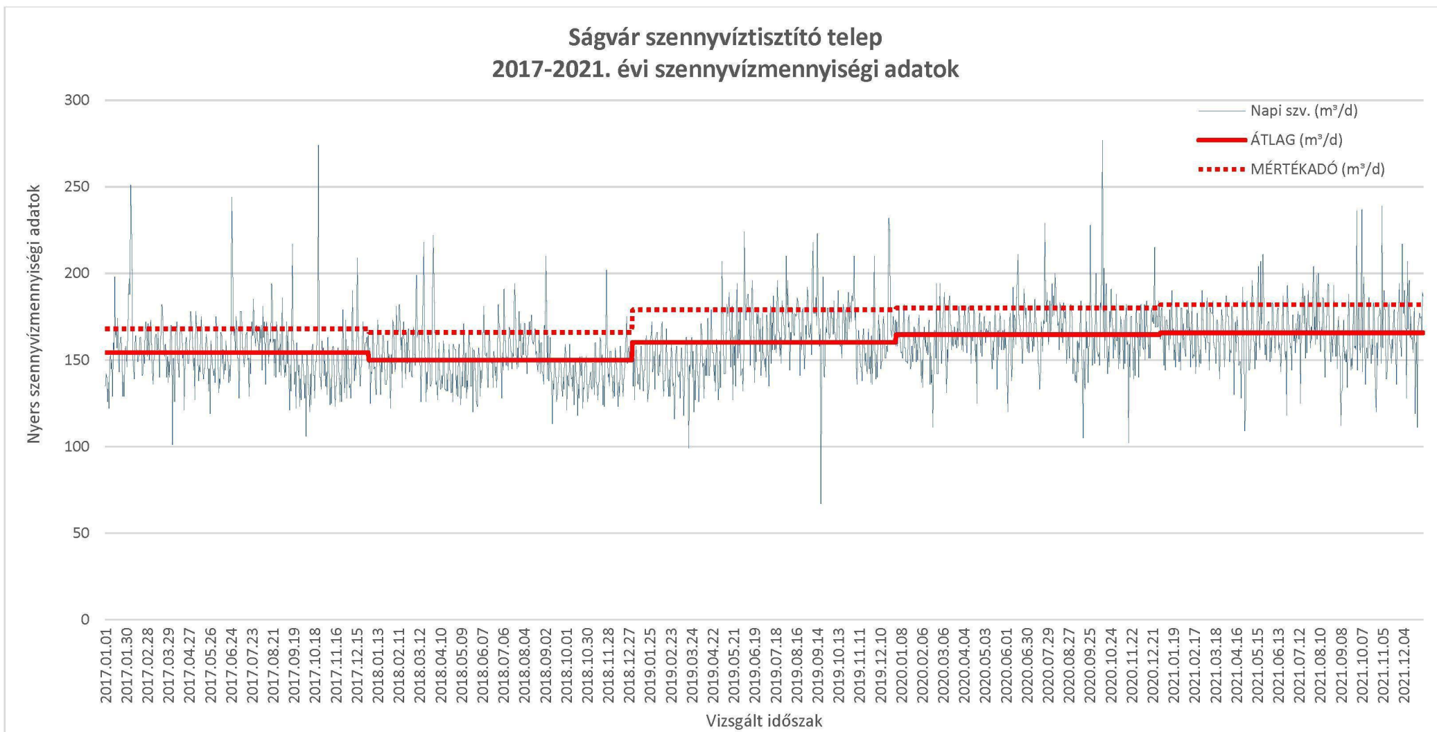
3.1. ábra_2017-2021. évi szennyvízmennyiségi adatok
